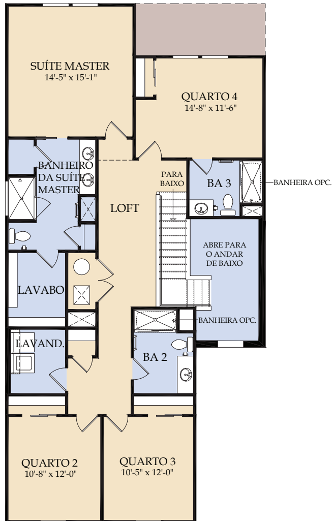
Segundo andar
