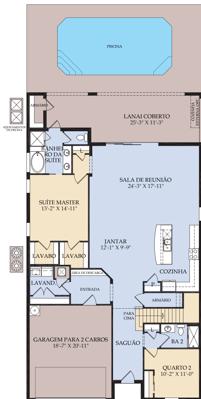
Primeiro andar
