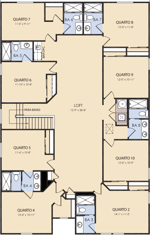
Segundo andar
