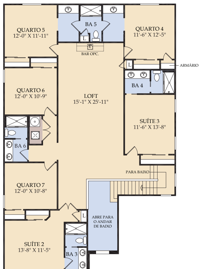
Segundo andar
